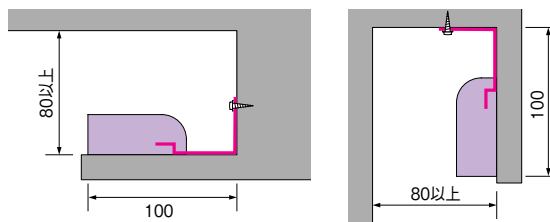
<L型金具使用例>
